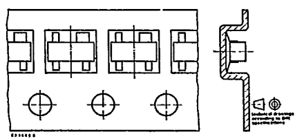
Fig. 7.5. Standard taped SOT 143
